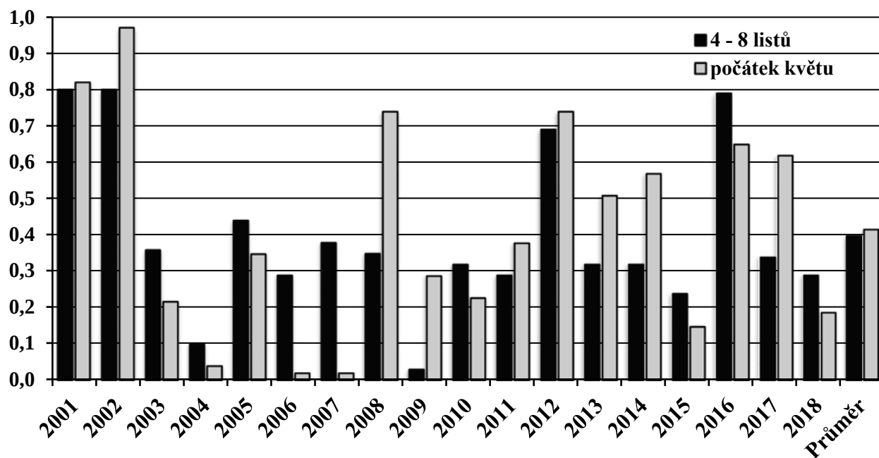
Graf 9: Průměrný přírůstek výnosu vztažený na kontroly (v t/ha, PP SPZO 2001 - 2018, pozemní aplikace)
