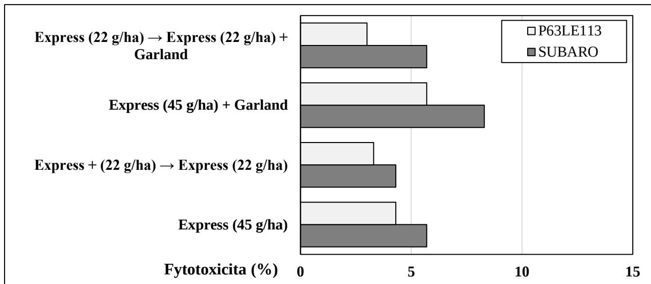
Graf 7: Průměrná fytotoxicita ExpressSun® technologie u vybraných hybridů v roce 2019 v pokusech ČZU Praha
