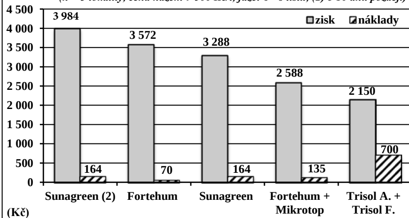
Graf 13: Náklady a zisk - stimulanty růstu a listová hnojiva - 2007 (n = 3 lokality, cena nažek: 9 500 Kč/t, fáze: 6 - 8 listů, (2) o 10 dnů později)
