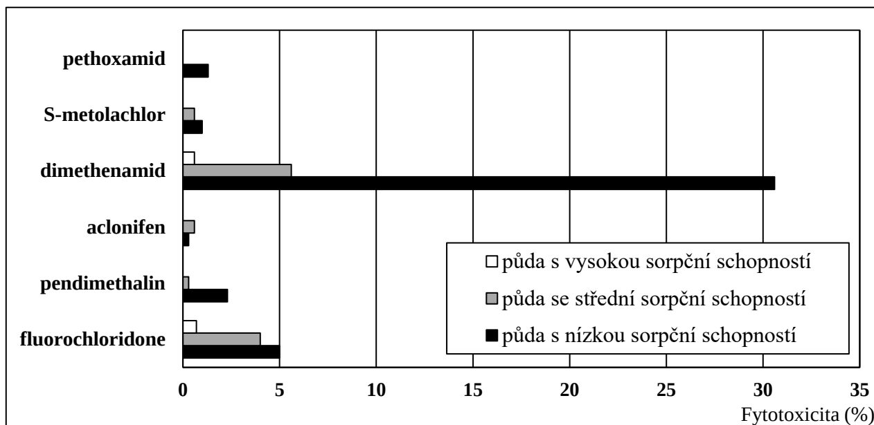
Graf 1: Selektivita testovaných herbicidů, průměrné výsledky z let 2015-2017, lokalita Praha, hlinitá půda, černoze (zdroj: prof. Ing. M. Jursík, Ph.D., ČZU Praha)
