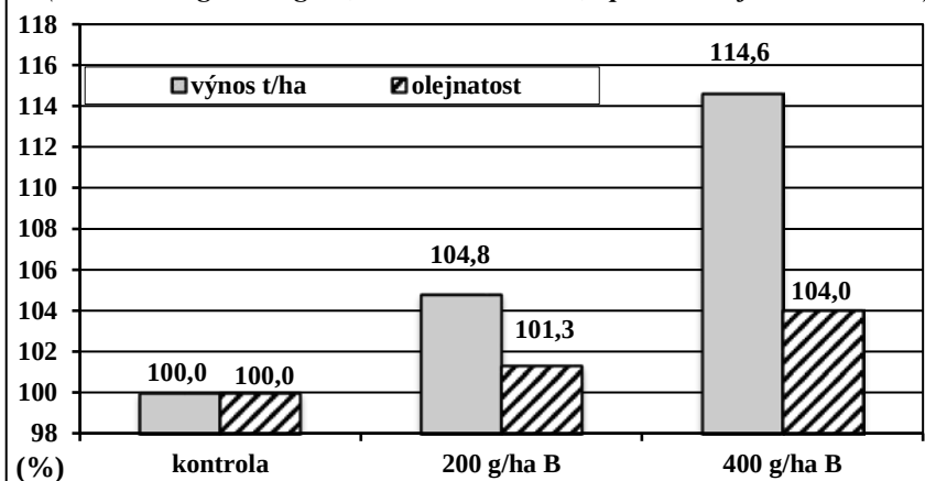
Graf 18: Vliv hnojení bórem na výnos slunečnice v % (dávka: 200 g a 400 g/ha, víceleté PP SPZO, aplikace ve fázi: 6 - 8 listů)
