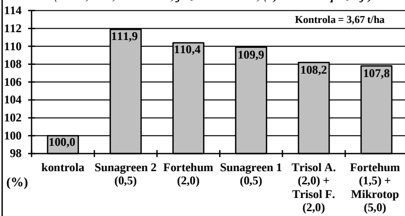
Graf 12: Průměrné hodnoty - stimulanty růstu a listová hnojiva - 2007 (n = 3, v %, PP SPZO, fáze: 6 - 8 listů, (2) o 10 dnů později)
